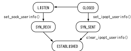
図 6 TCP 状態遷移と USERINFO の操作 Fig. 6 TCP state transition and manipulation USERINFO
