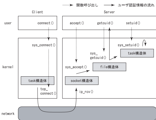
図 5 システムの概要 Fig. 5 Overview of the system
